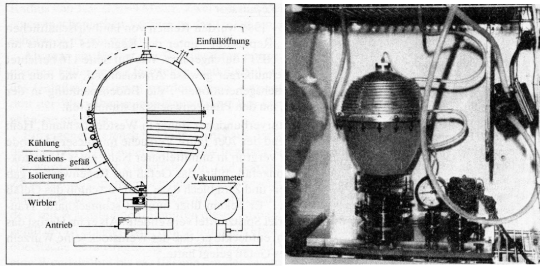
Bild 18 Aufbau der „Repulsine“ nach Viktors Angaben [1]
