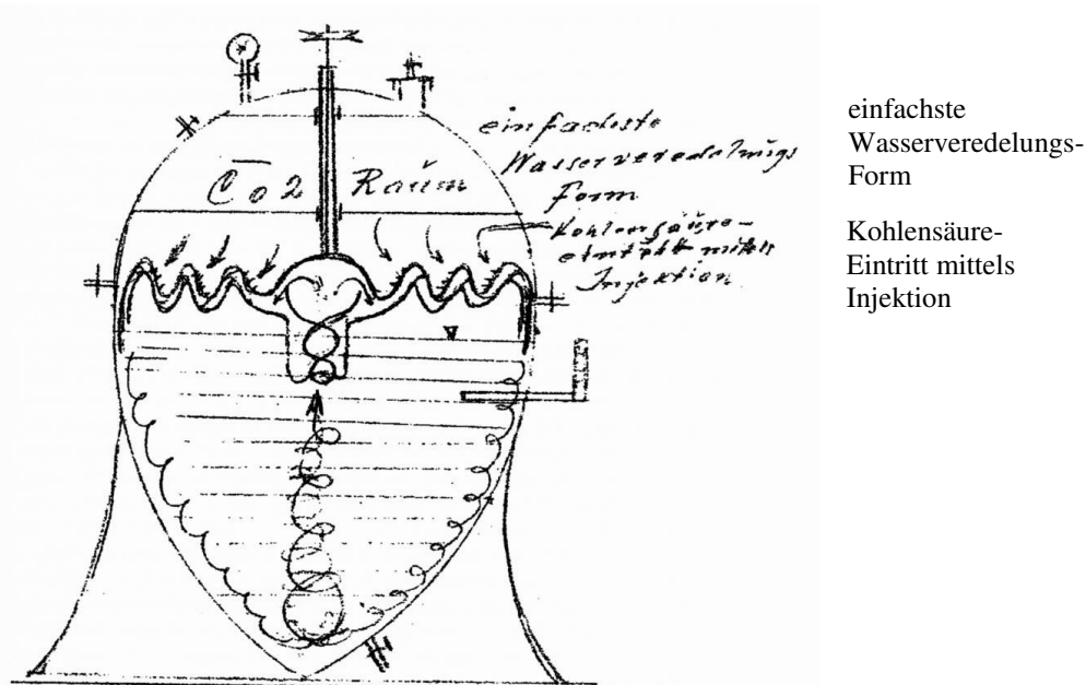
Bild 12 Viktors Skizze eines Geräts zur Wasserveredelung mit Verbundwirbel
