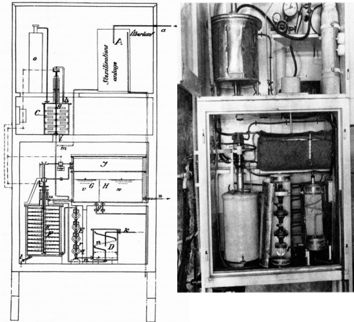
Bild 4 Patentiertes Edelwasser-Gerät [2]
